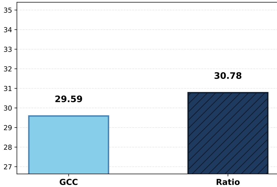
VMAF
