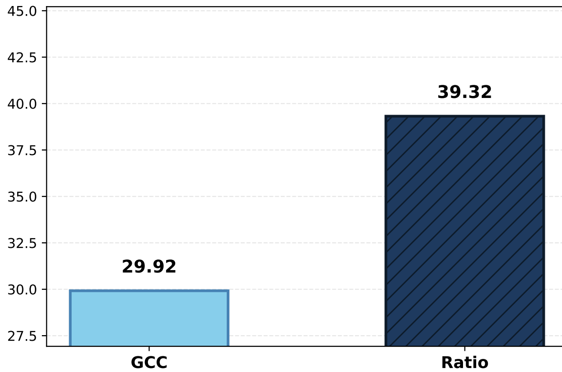
VMAF
