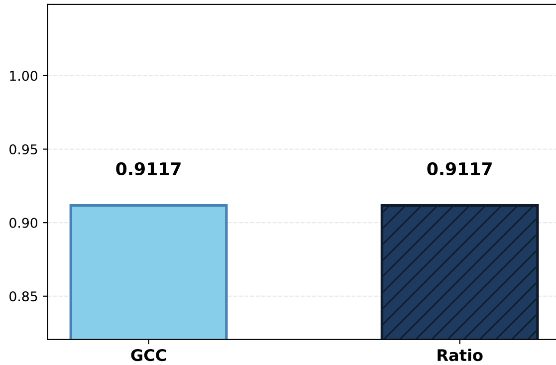
LPIPS
