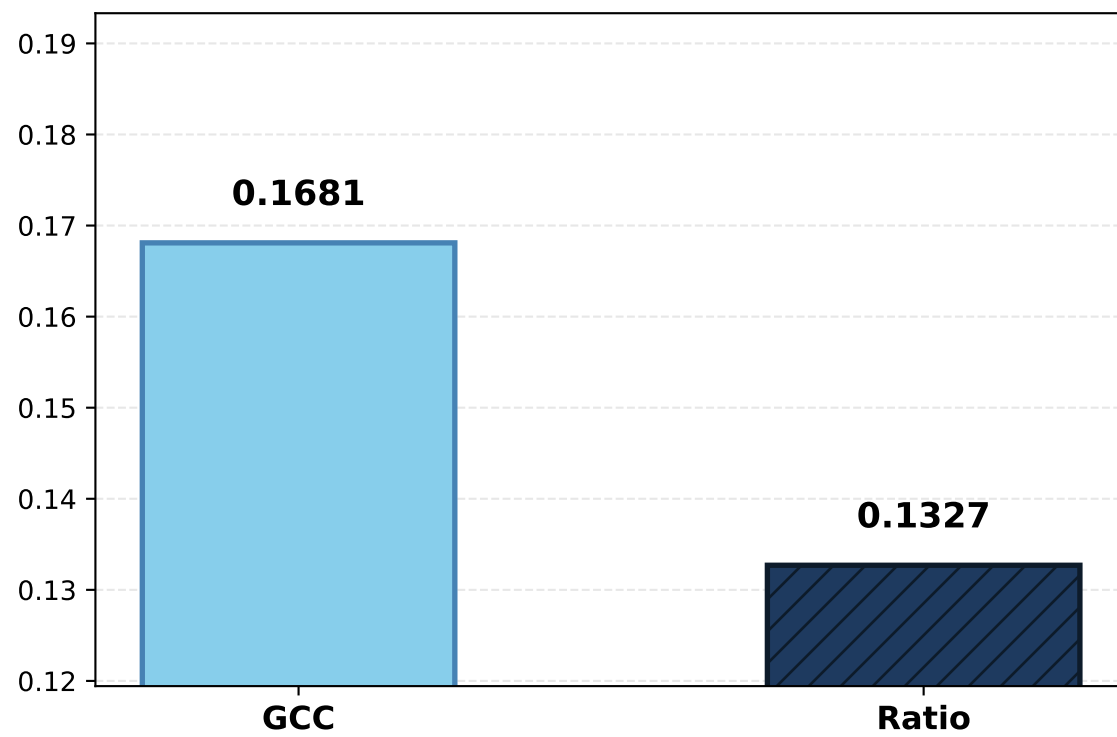
LPIPS
